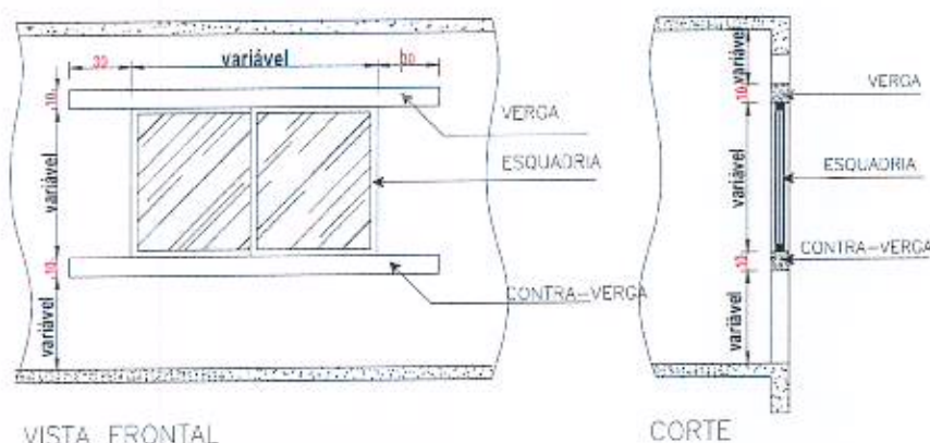
DETALHE-03 VERGAS E CONTRA-VERGAS EM VÃOS DE PORTAS E JANELAS
